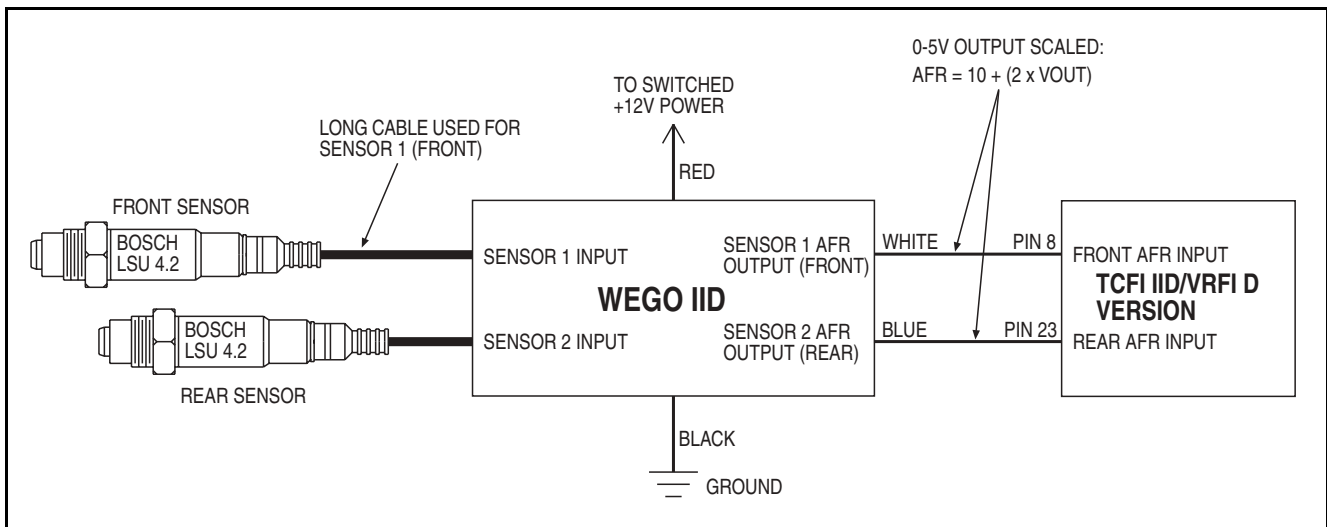
Figure 2 - WEGO Hookup
